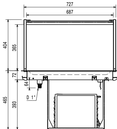
Front aanzicht
