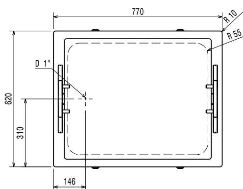
Boven aanzicht
